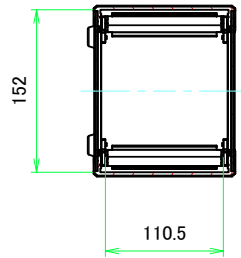
A-A (1:5)
